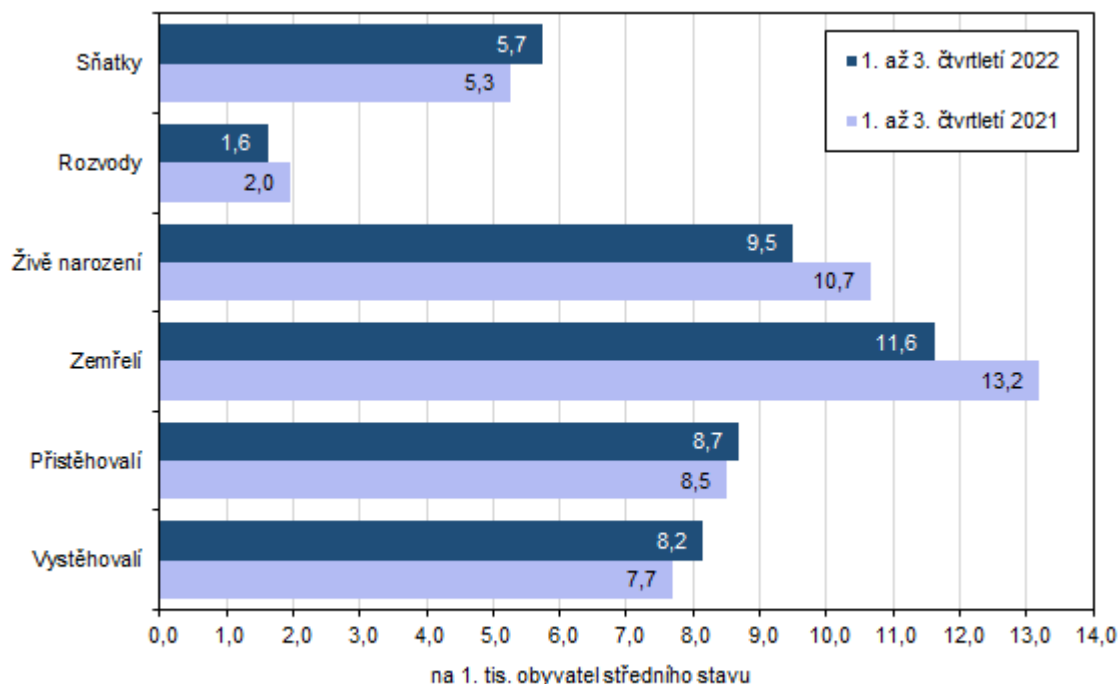
Graf 1 Pohyb obyvatelstva ve Zlínském kraji v 1. až 3. čtvrtletí 2021 a 2022
