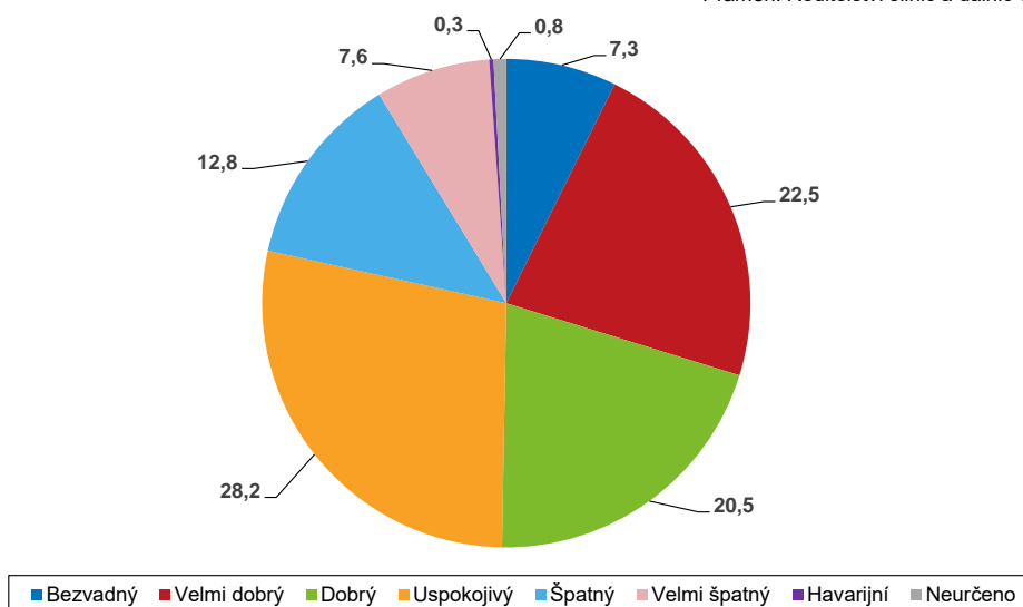
Mosty podle stavu nosné konstrukce nebo spodní stavby v Ústeckém kraji k 1. 1. 2023
