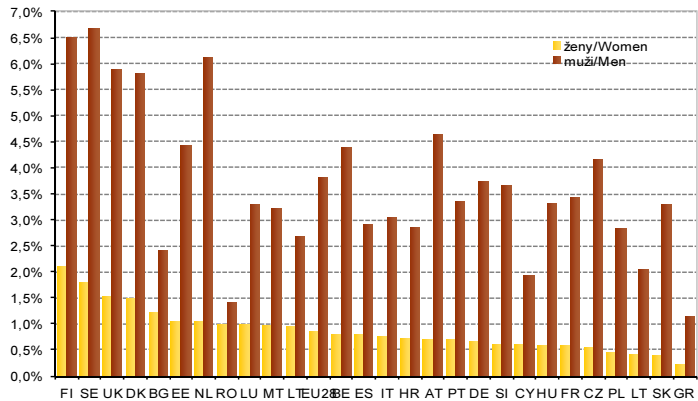
Graf 13: Podíl IT odborníků na zaměstnané populaci podle pohlaví, 2015 IT professionals as a percentage of total employment in given sex, 2015
