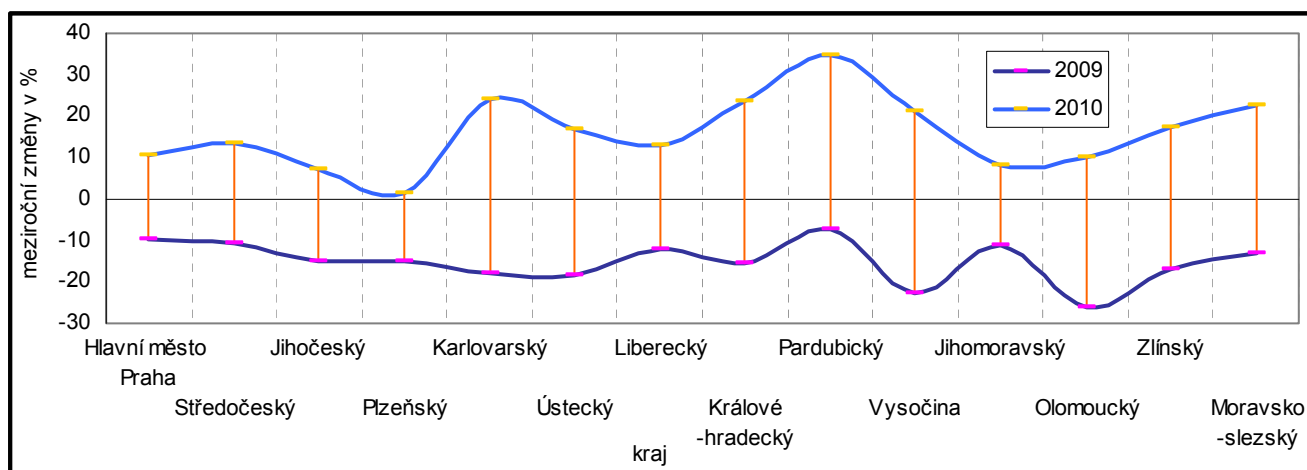
Graf 2 Meziroční změny vývozu krajů v roce 2009 a 2010
